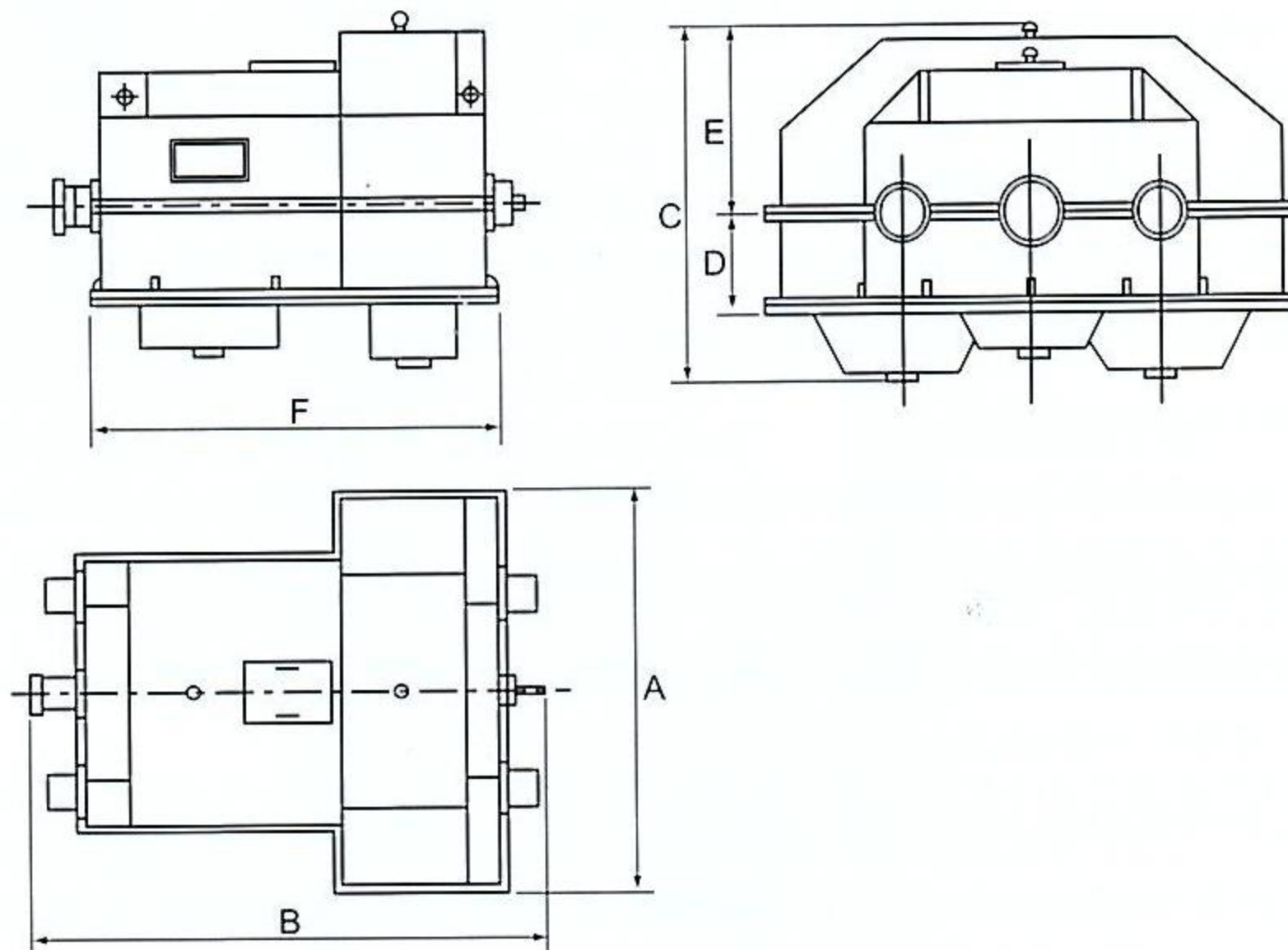
GMY 系列中心传动磨机减速机(二级)
