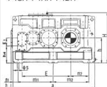
P4SH P4HH P4DH
