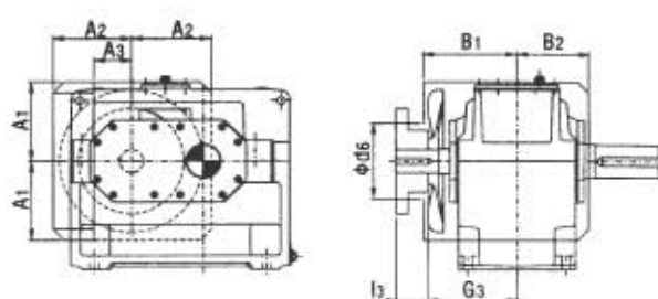
P1SH3 ... 11 冷却风扇/with fan
