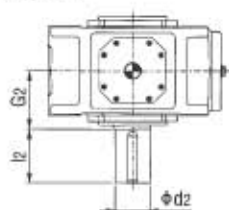
V3SV 实心轴 Solid shaft
