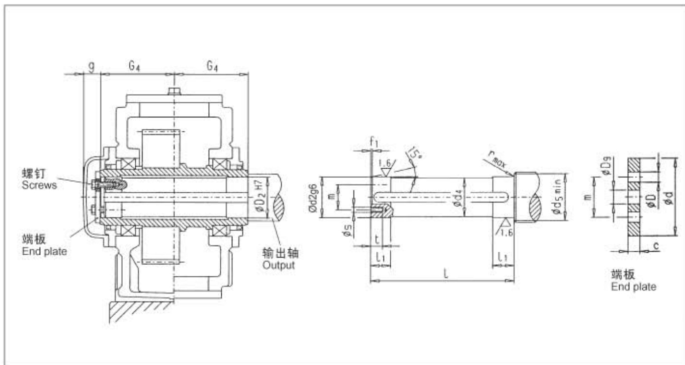
类型 /Types P2H.,P3H.,P4H.,V3H.,V4H.
