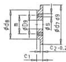
端板 End plate
