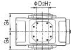
P2HV 空心轴 Hollow shaft
