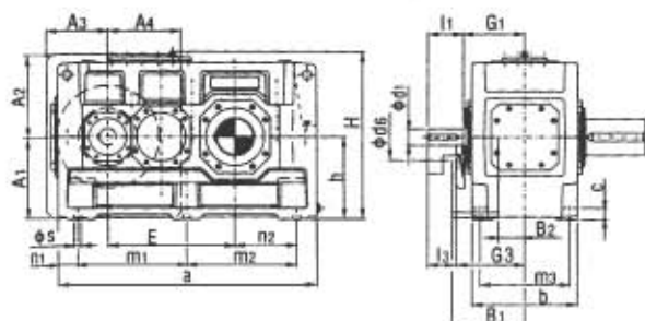
P2SH P2HH P2DH
