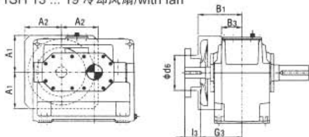
P1SH 13 ... 19 冷却风扇/with fan
