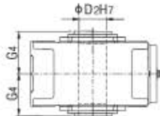
P3HV 空心轴 Hollow shaft
