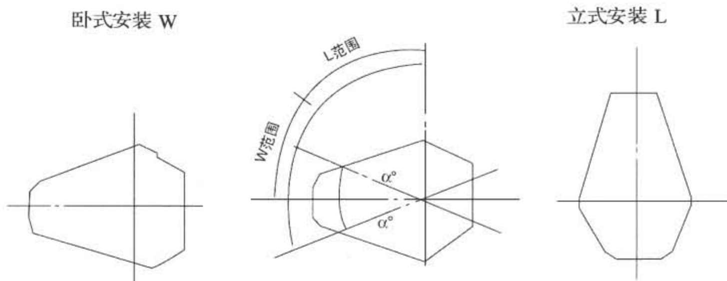
图2 减速器安装型式
