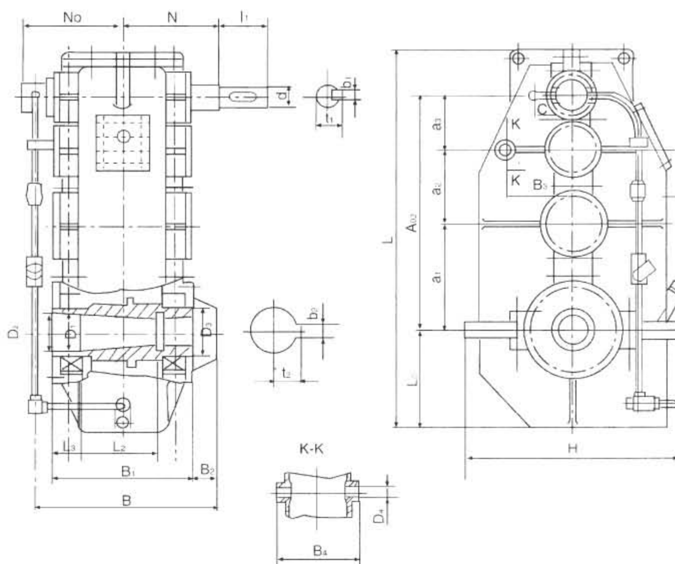
图14 QJ-T 型减速器外形及安装尺寸
