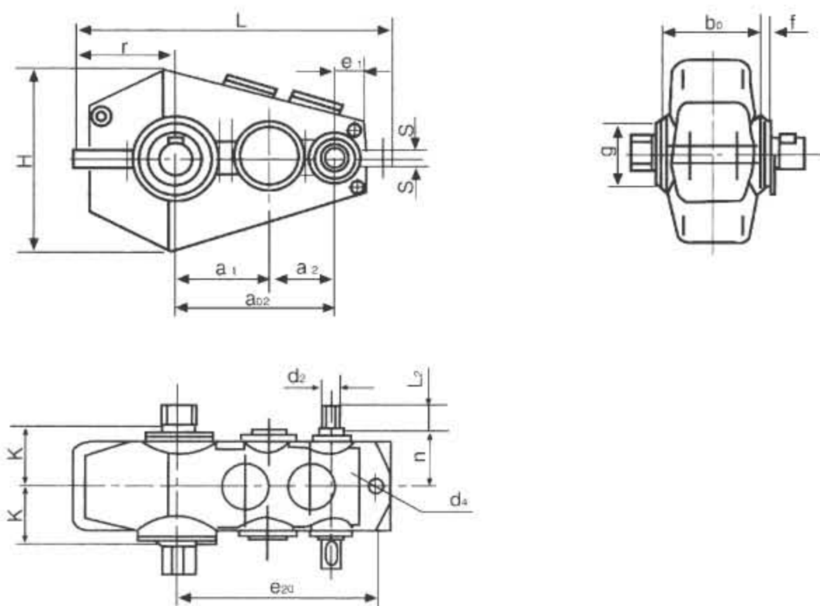
图5 QJR(QJB)减速器外形尺寸
