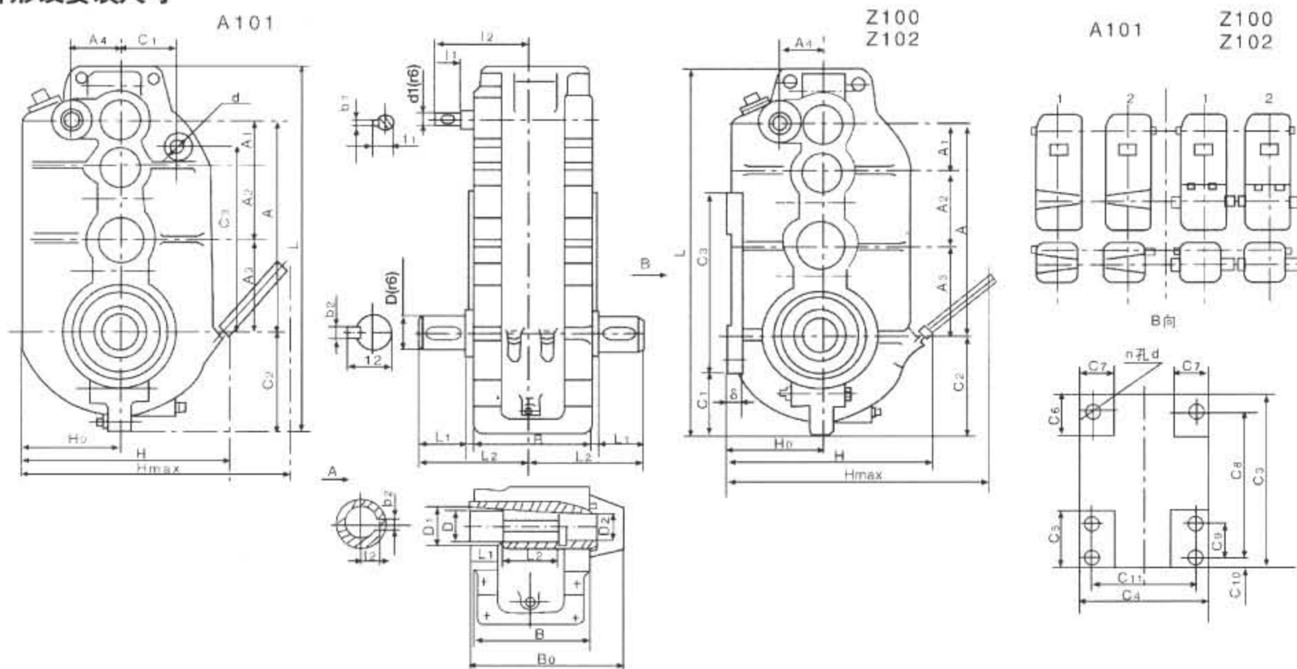
ZSC(D) 型大速比减速器
