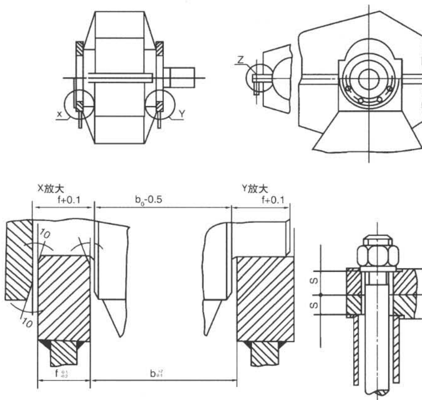
图3 减速器三支点支承型式
