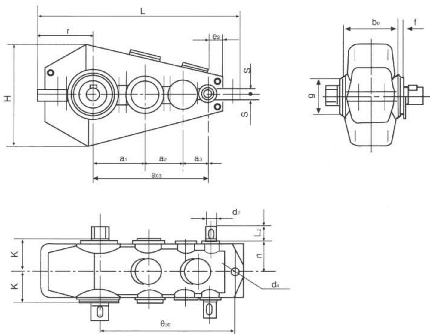
图6 QJS(QJC)减速器外形尺寸
