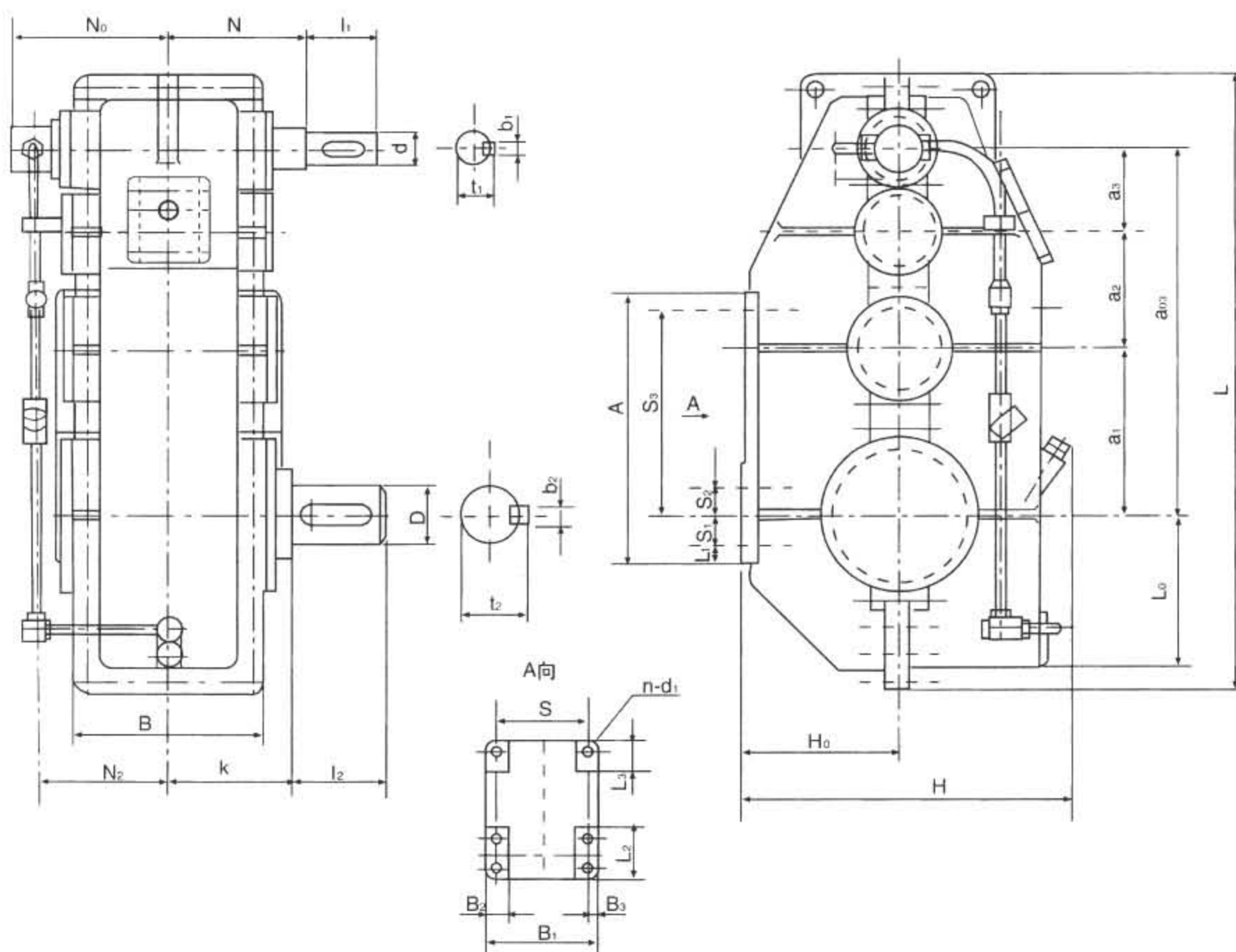
图12 QJ-L型减速器的外型及安装尺寸
