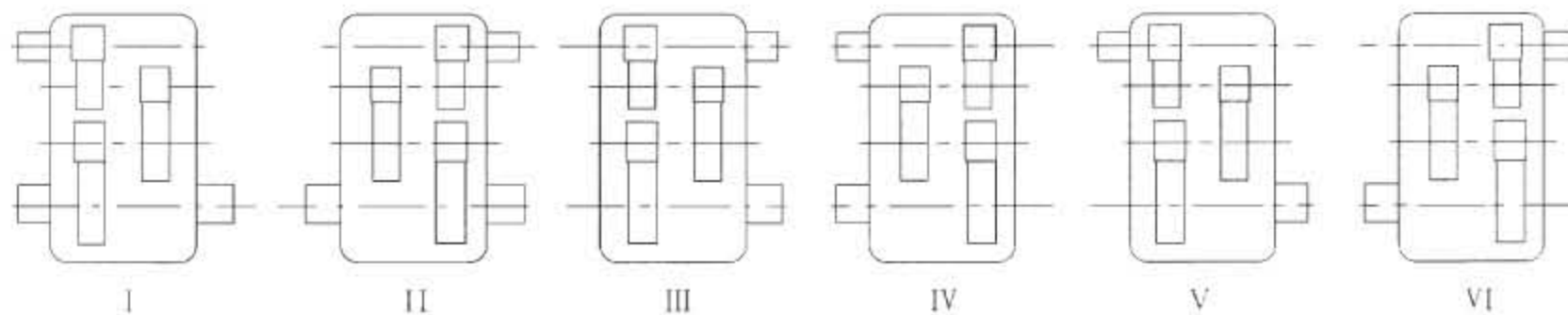
图11 QJ-L 型减速器装配形式
