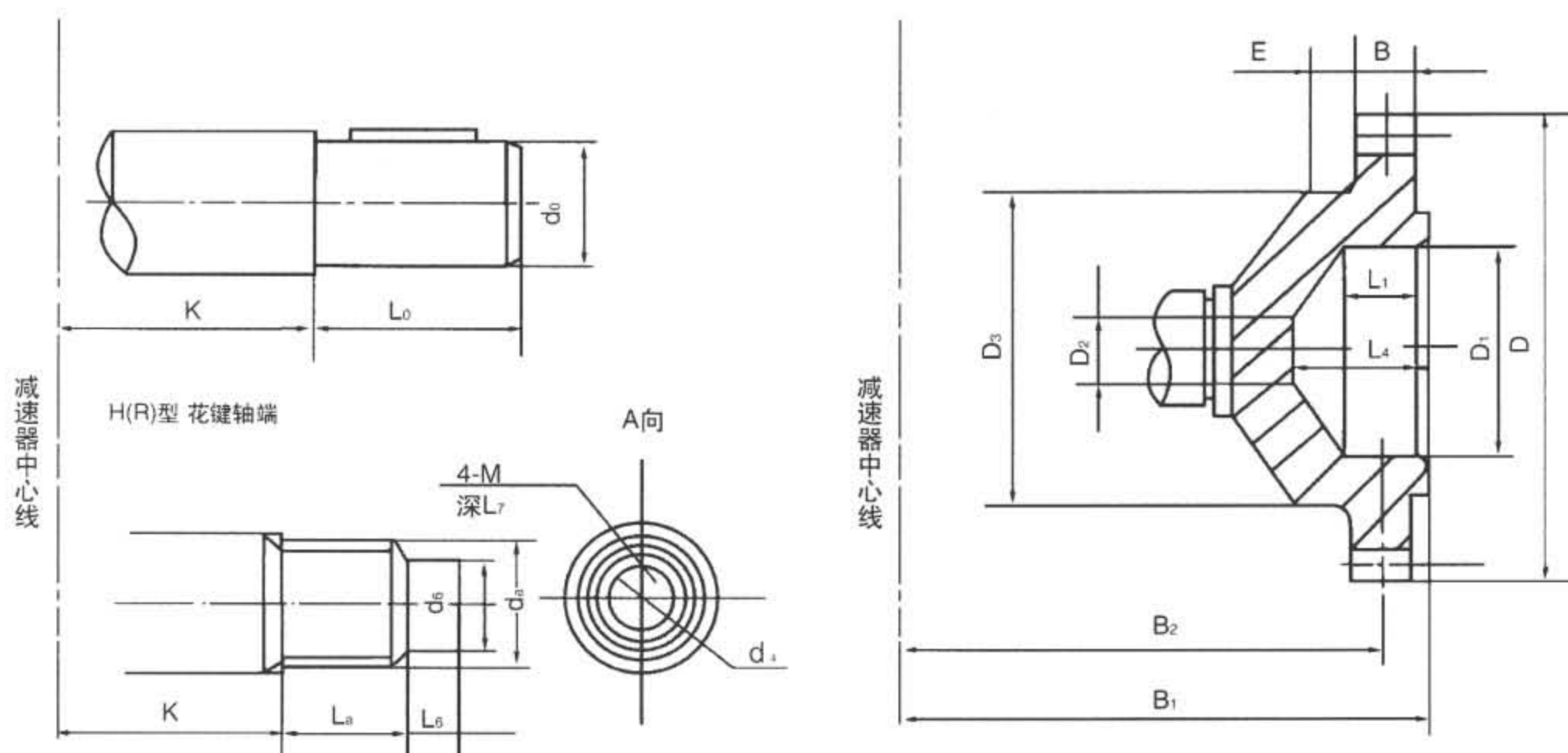
图4 输出轴端型式
