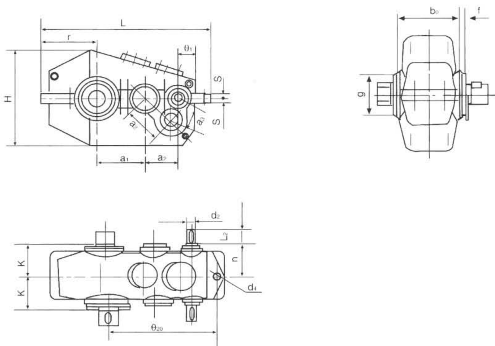
图7 QJRS(QJD)减速器外形尺寸
